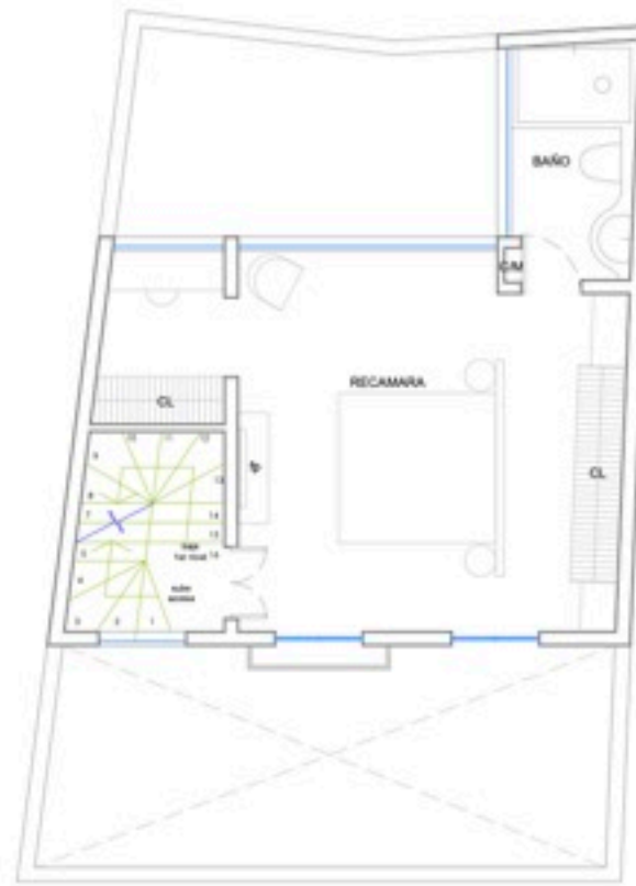
Esc: 1/75 Barranca 74 2do. nivel
