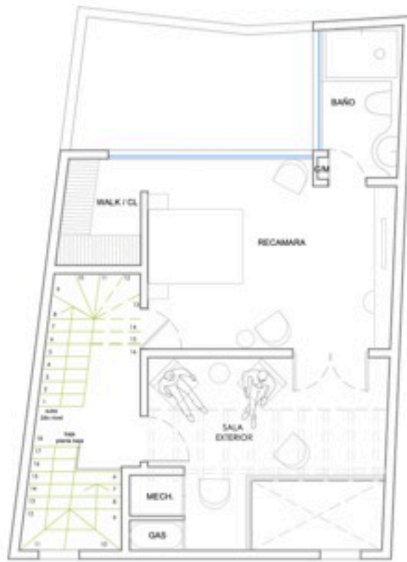
Esc: 1/75 Barranca 74 1er. nivel
